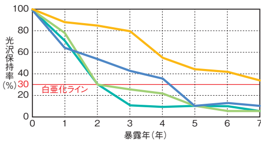
● 宮古島7年暴露における耐候性比較
