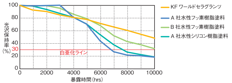
● 促進耐候性試験 (XWOM)
