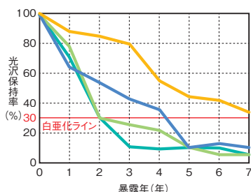
●宮古島7年暴露における耐候性比較
