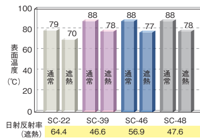
赤外ランプにおける塗膜表面温度 (500 W)
