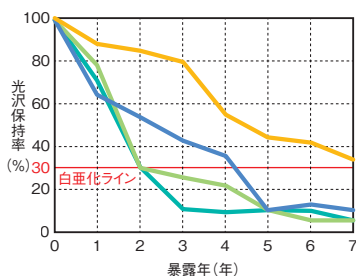
●宮古島7年暴露における耐候性比較
