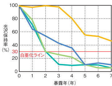
●宮古島7年暴露における耐候性比較
